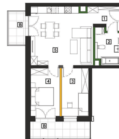
Rzut w skali 1:200
