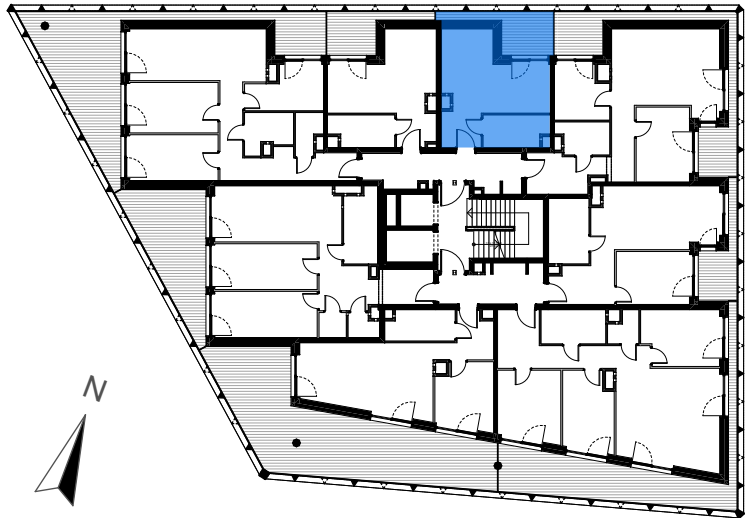
PIĘTRO 5 MIESZKANIE A.35
