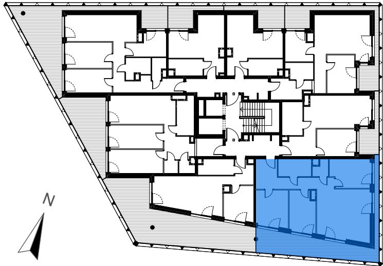
PIĘTRO 4 MIESZKANIE A.30
