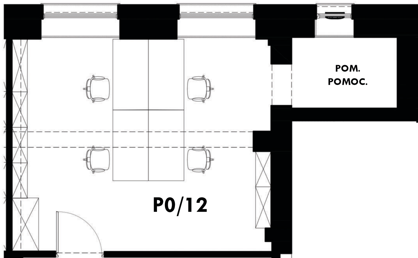
SCHEMAT LOKALIZACYJNY
